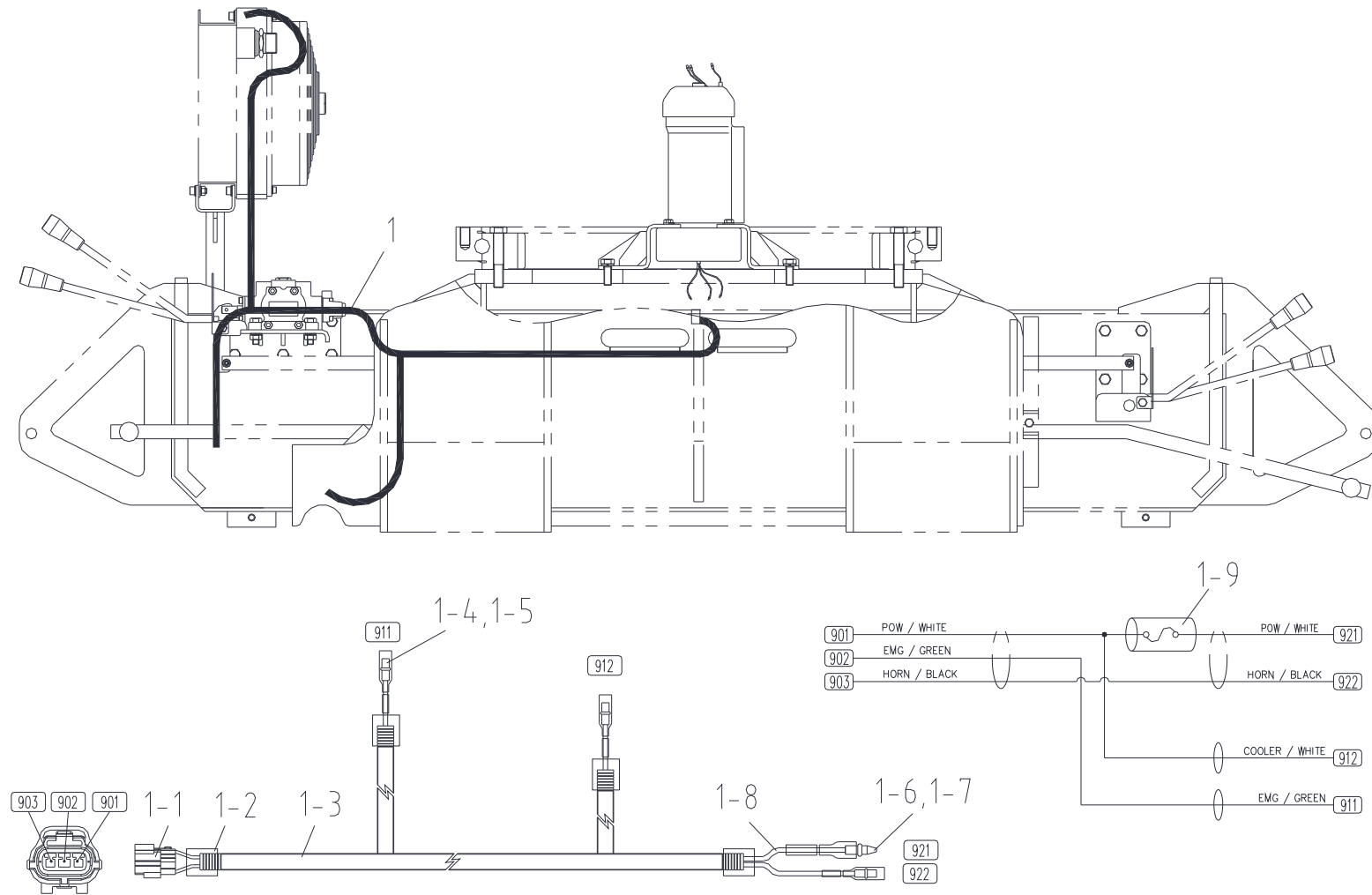
프레임 전선 Fig. 10-1 SCS876 FRAME WIRING
