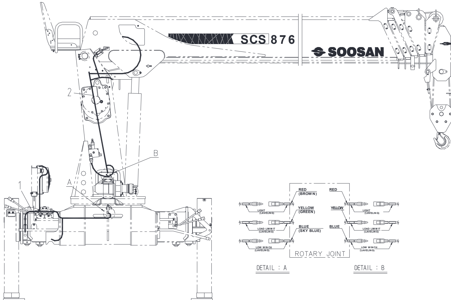
전선 조립체 Fig. 10 SCS876 WIRING ASS'Y
