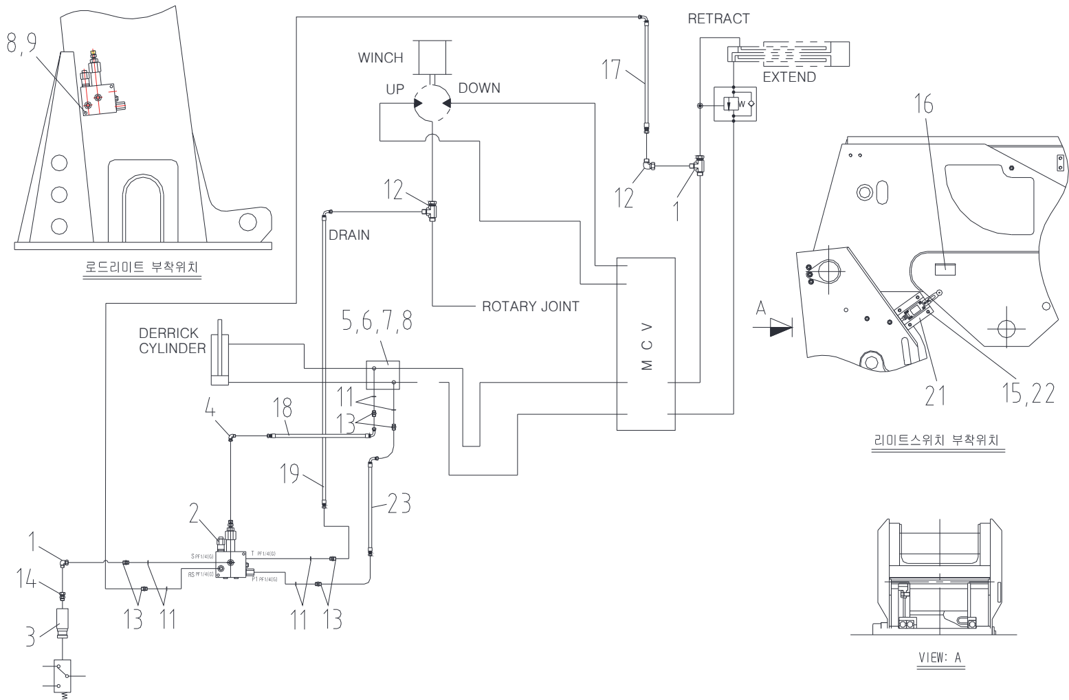
과하중방지 배관 조립체 Fig. 5-7 SCS876 OVERWINDING ALARM PIPING ASS'Y
