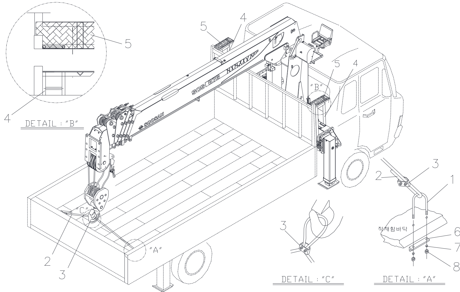
로딩 박스 파트 Fig. 9-5 SCS876 LOADING BOX PART
