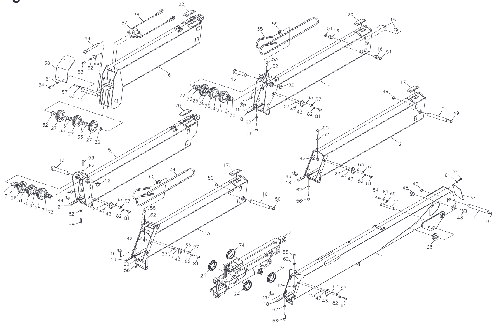
붐 조립체 Fig. 1 SCS876 BOOM ASS'Y
