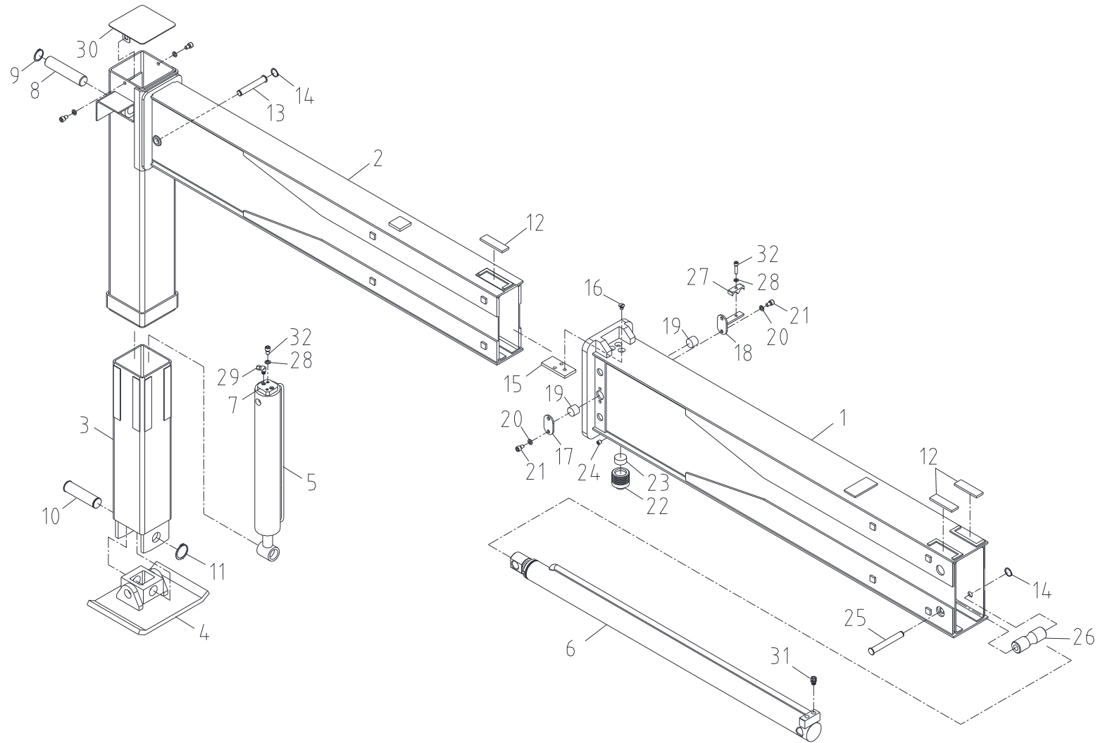
아우트리거 조립체 Fig. 4 SCS876 OUTRIGGER ASS'Y
