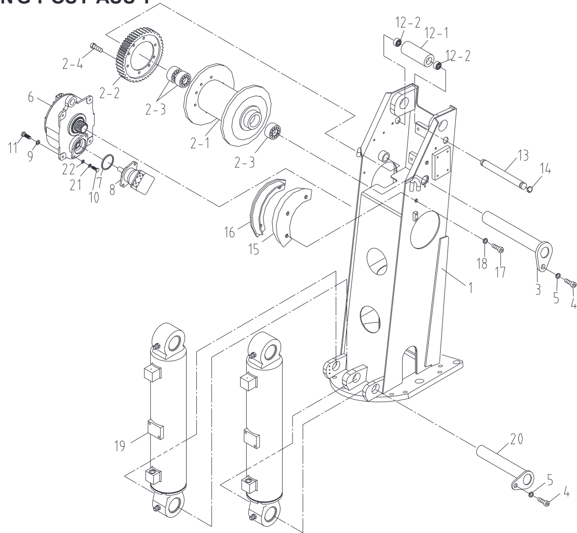
스윙 포스트 조립체 Fig. 2 SCS876 SWING POST ASS'Y
