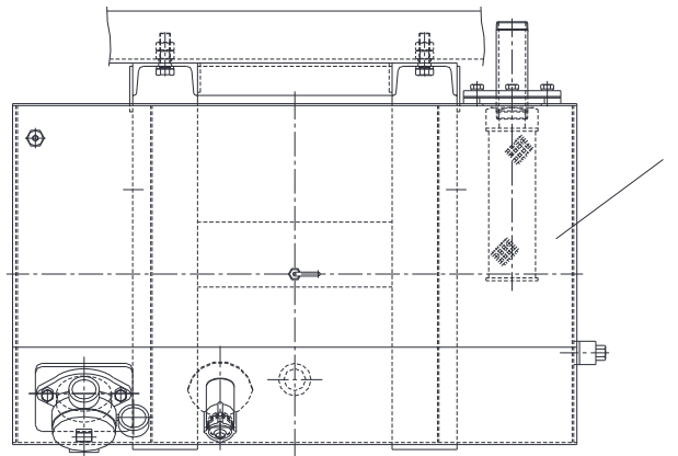
오일 탱크 셋트 Fig. 9-6-1 SCS876 OIL TANK SET
