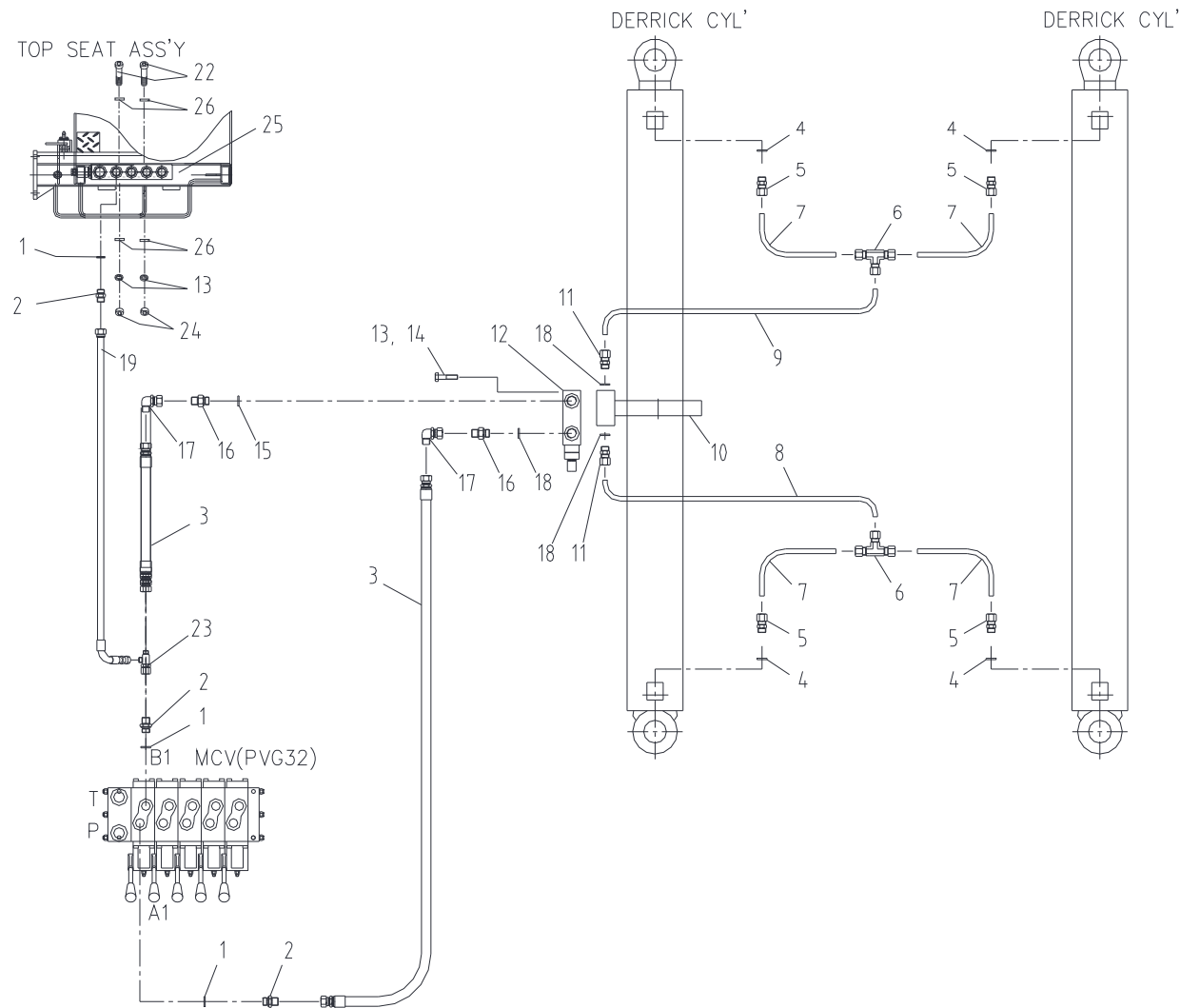
데릭 배관 Fig. 5-2 SCS876 DERRICK PIPING
