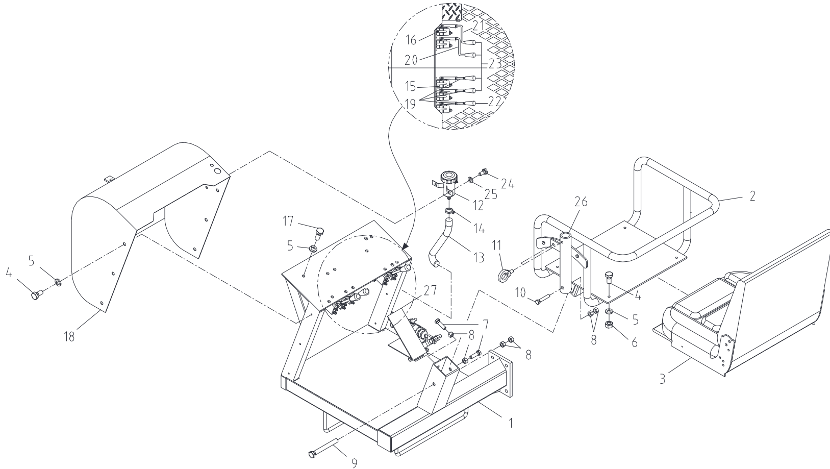
탑 시트 조립체 Fig. 8 SCS876 TOP SEAT ASS'Y
