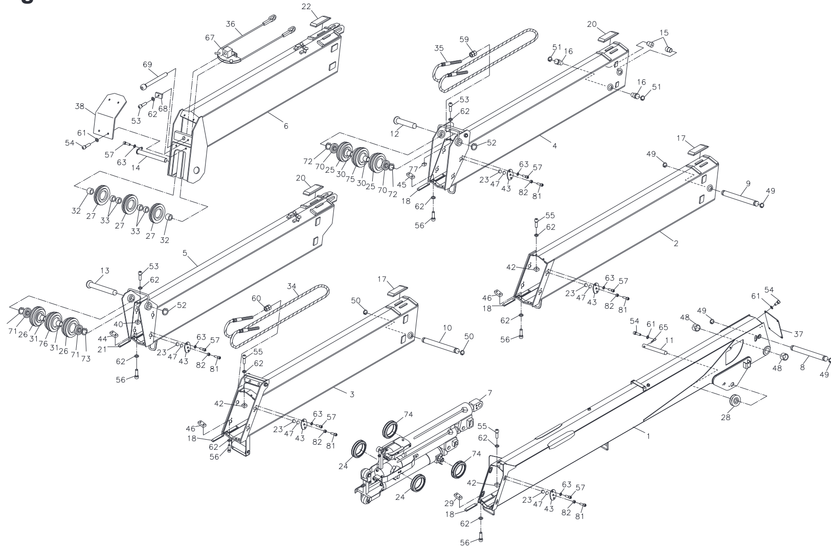
붐 조립체 Fig. 1 SCS876 BOOM ASS'Y
