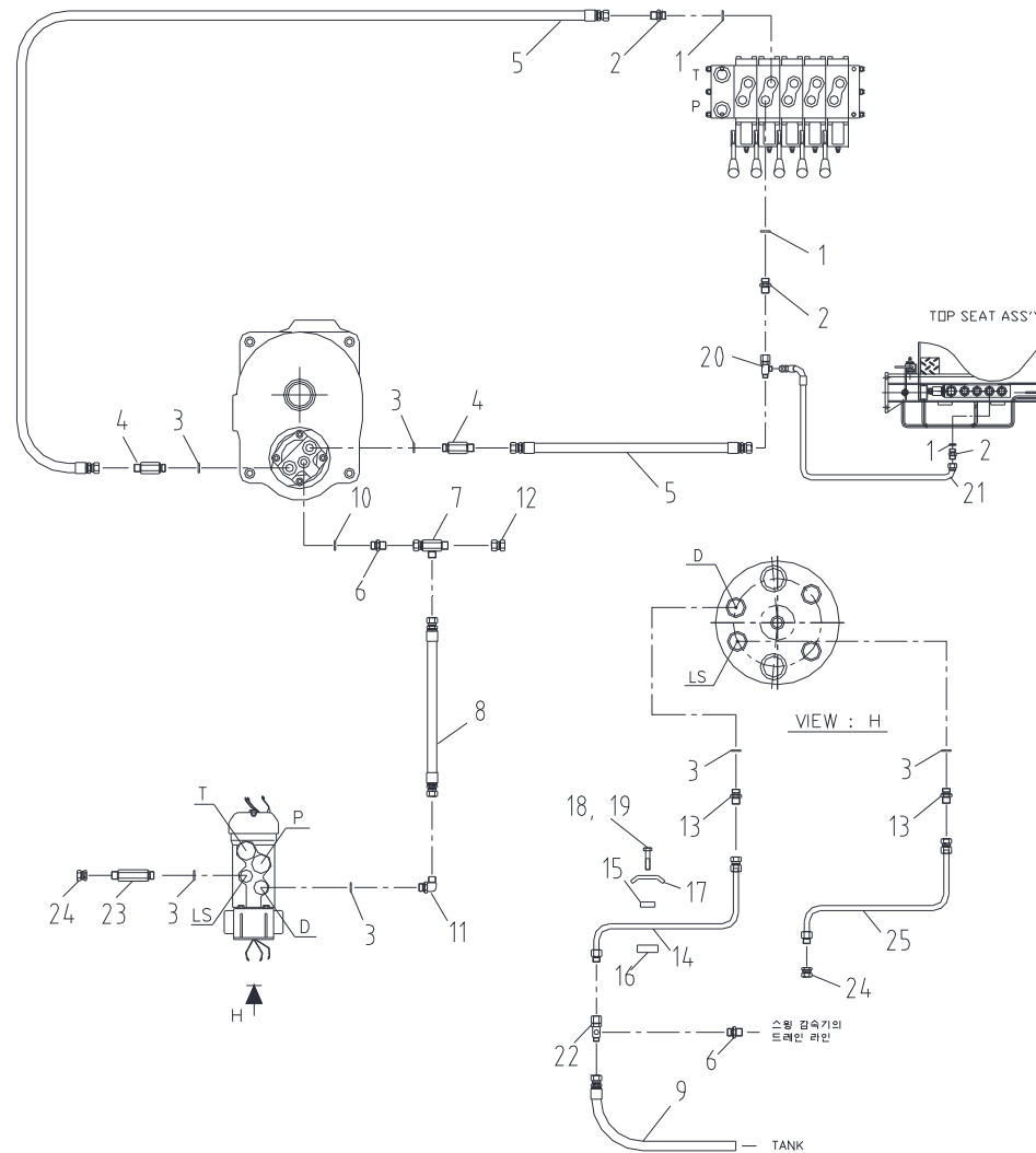
메인 윈치 배관 Fig. 5-3 SCS876 MAIN WINCH PIPING
