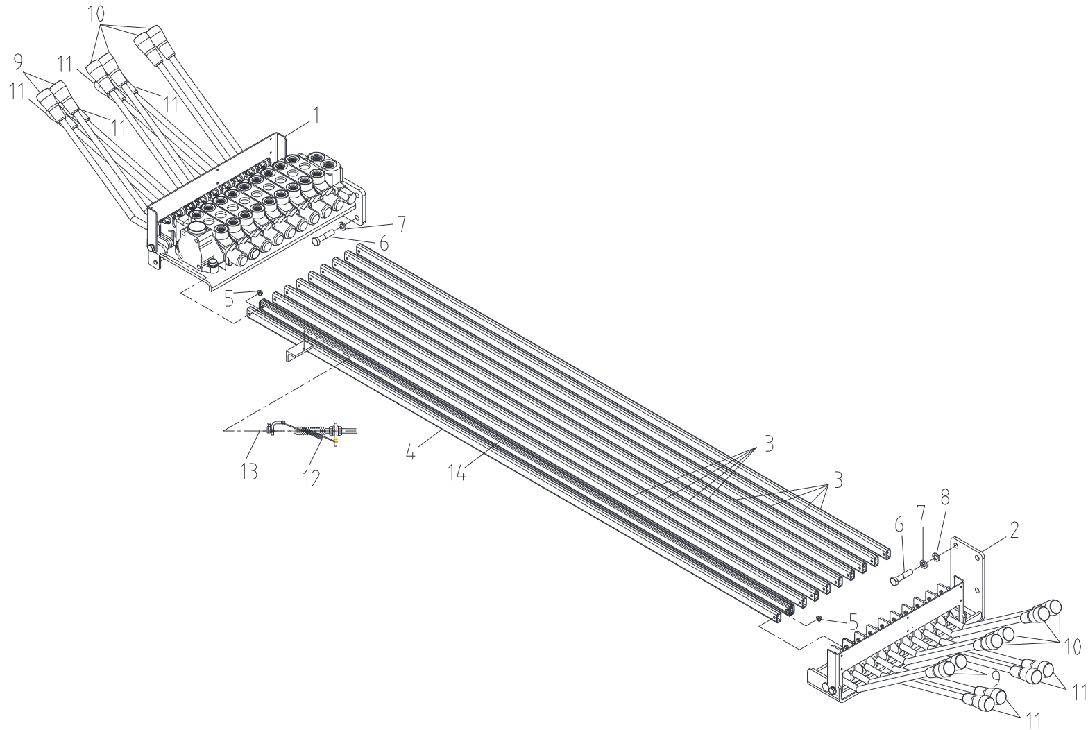
오퍼레이션 조립체 Fig. 3-2 SCS876 OPERATION ASS'Y
