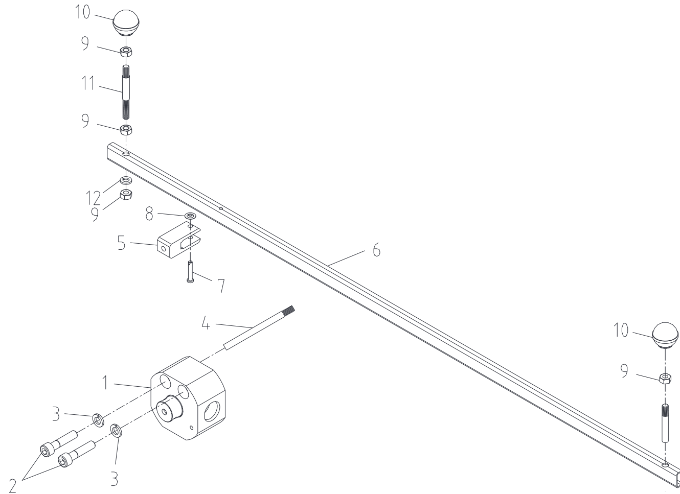
디버터 밸브 셋 Fig. 3-3 SCS876 DIVERter V/ V SET
