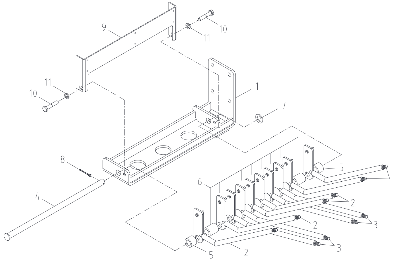
레버 스텐드 세트 Fig. 3-2-2 SCS876 LEVER STAND SET
