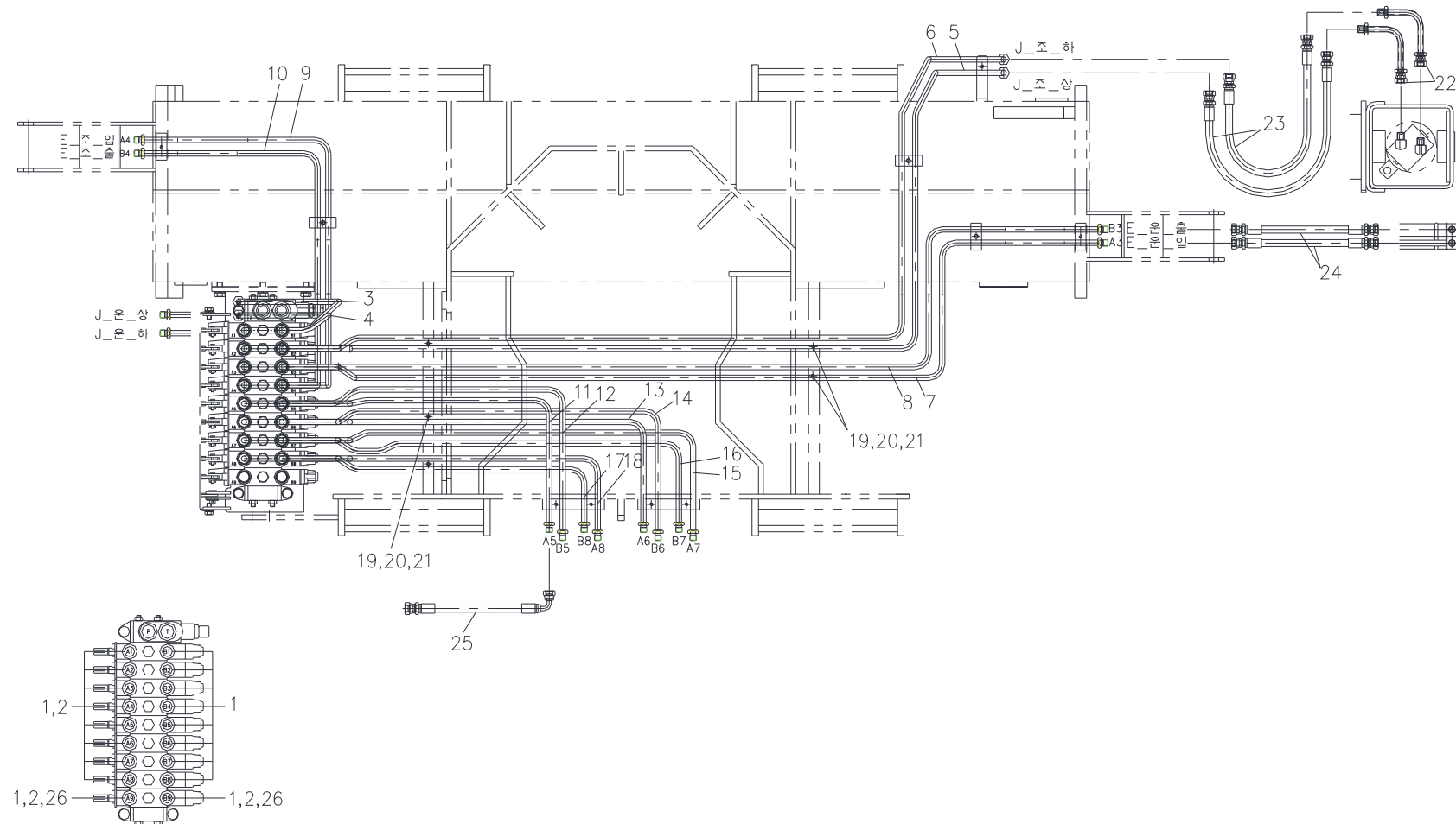
아우트리거 배관 Fig. 5-6 SCS876 OUTRIGGER PIPING
