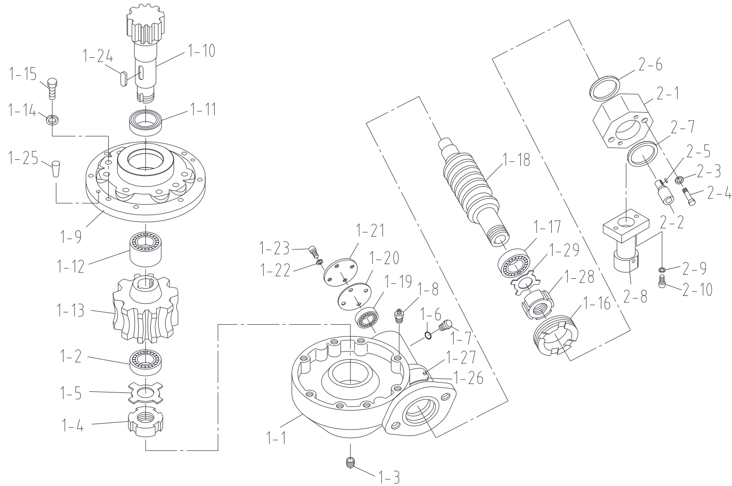
스윙 감속기 세트 Fig. 2-3 SCS876 SWING R/ G SET
