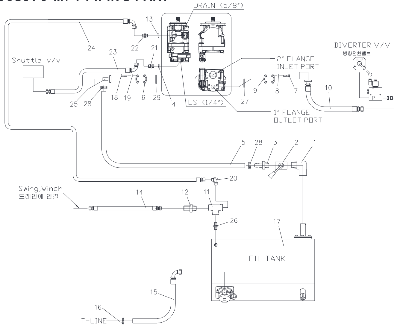
장착 배관 파트 Fig. 9-6 SCS876 M/ T PIPING PART
