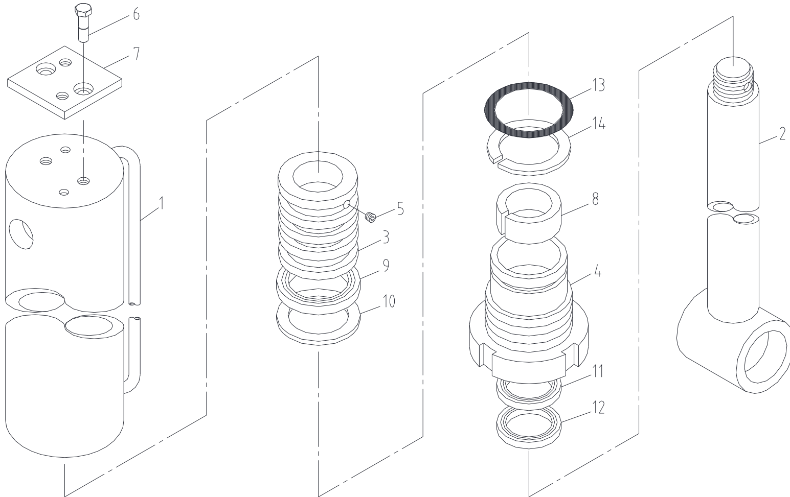
잭 실린더 조립체 Fig. 4-1 SCS876 JACK CYL' ASS'Y
