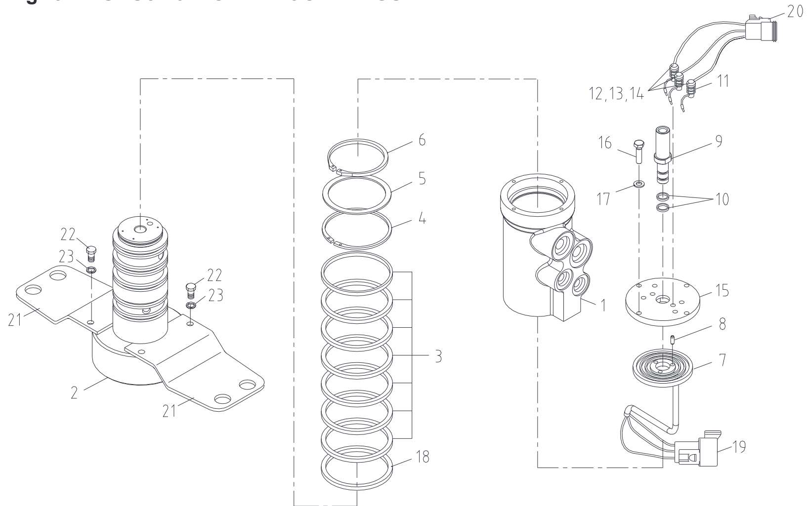
로타리 조인트 조립체 Fig. 3-1 SCS876 ROTARY JOINT ASS'Y
