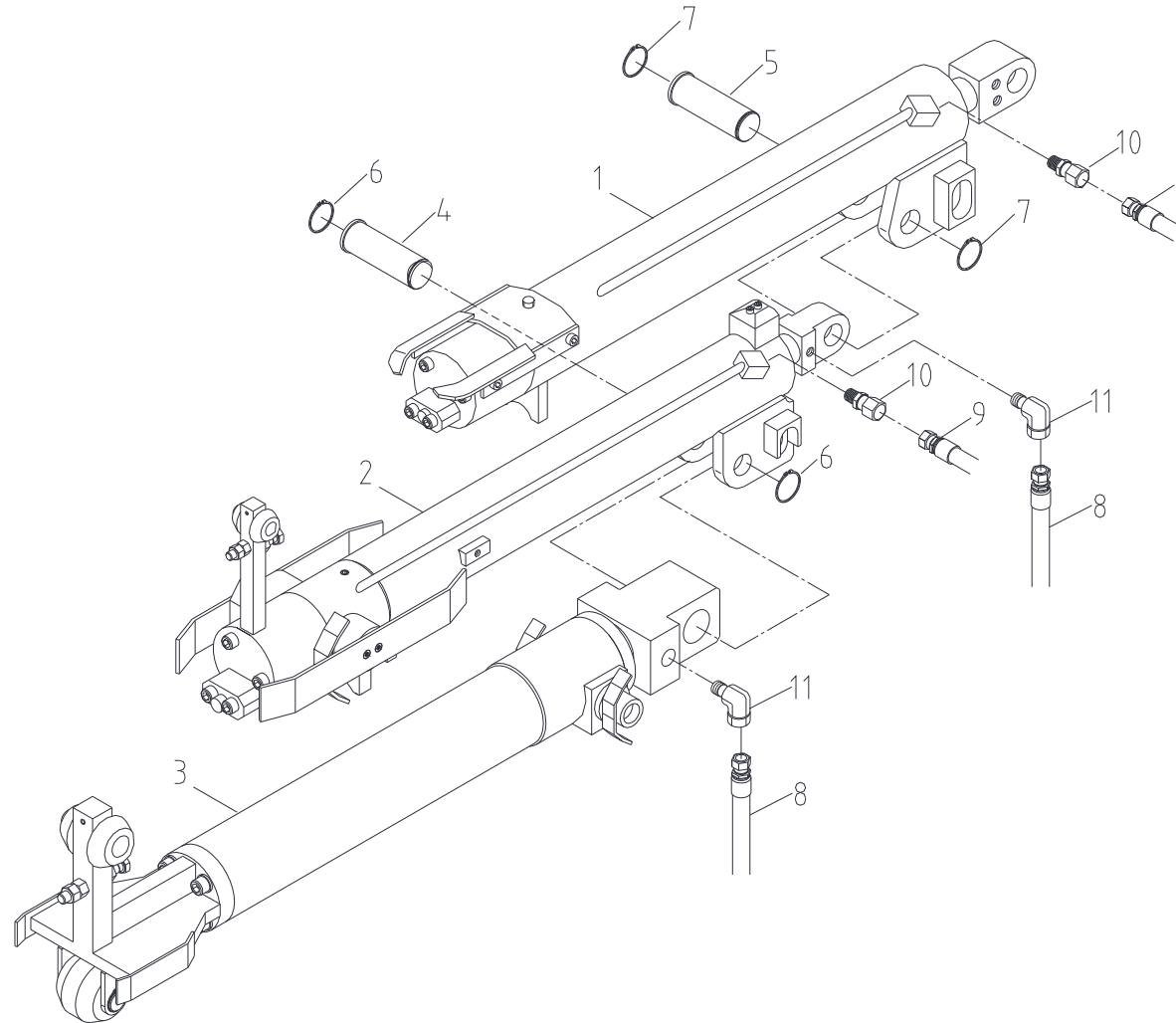
텔레스코픽 실린더 조립체 Fig. 1-1 SCS877 TELESCOPIC CYL' ASS'Y
