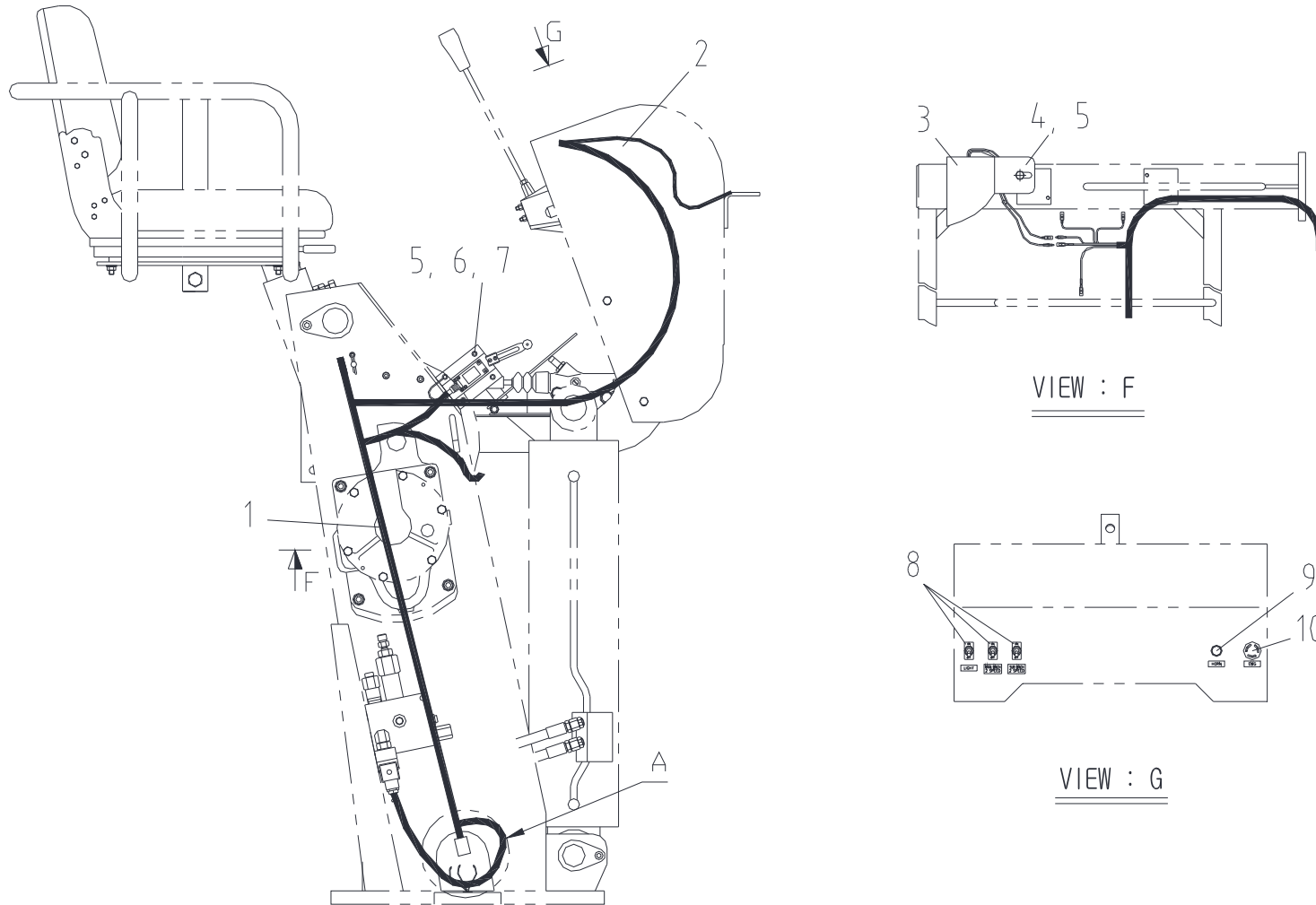
포스트 전선 Fig.10-2 SCS876 POST WIRING
