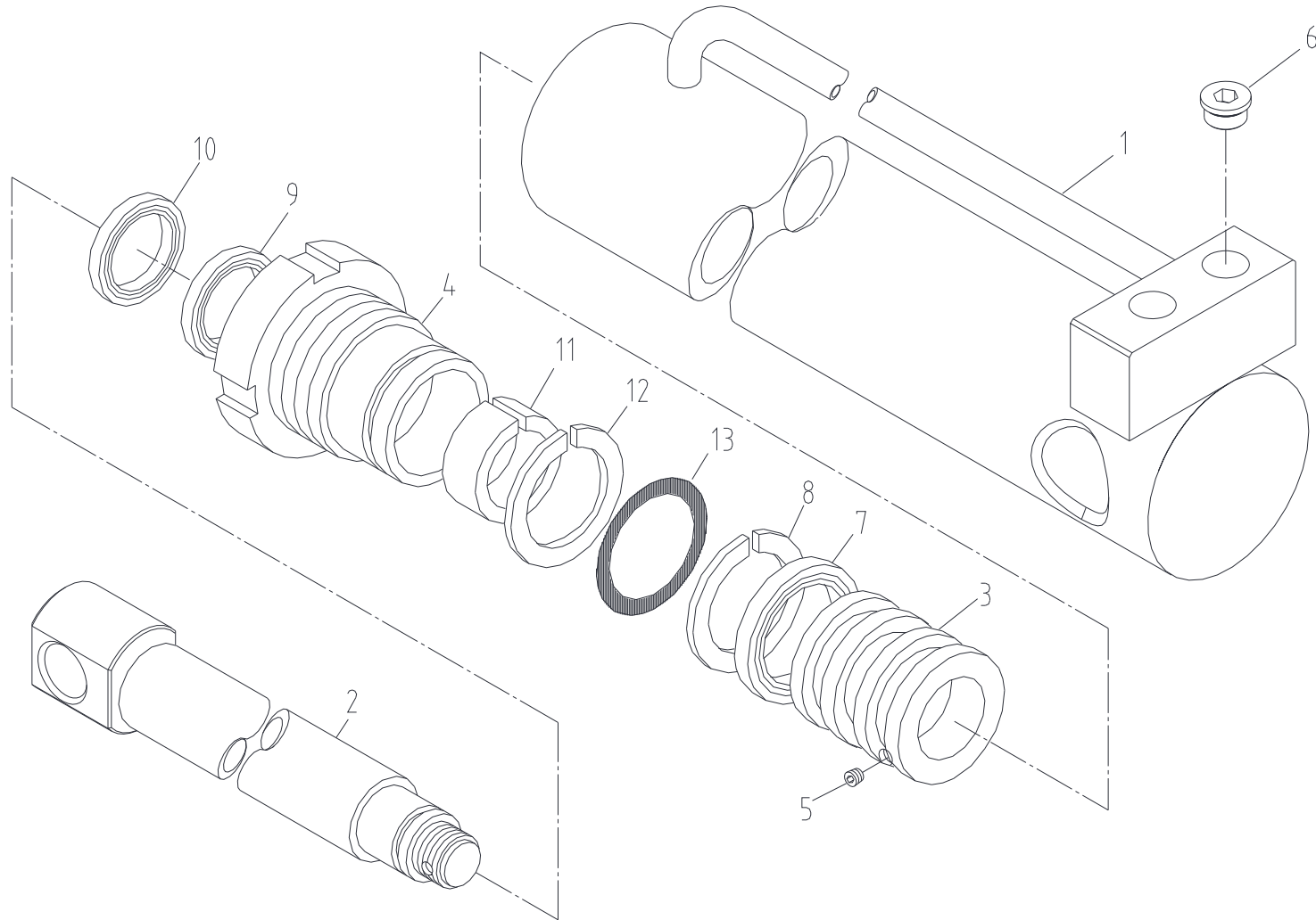
익스펜딩 실린더 조립체 Fig. 4-2 SCS876 EXPANDING CYL' ASS'Y
